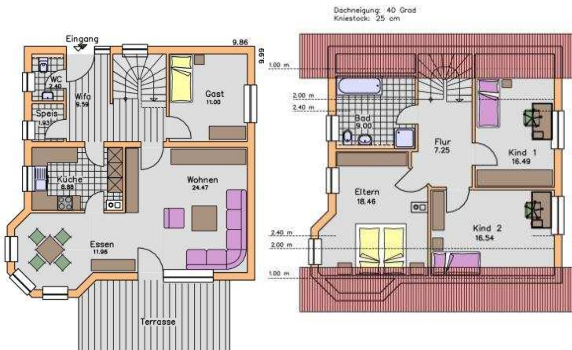
Grundriss EG 68 m 2
